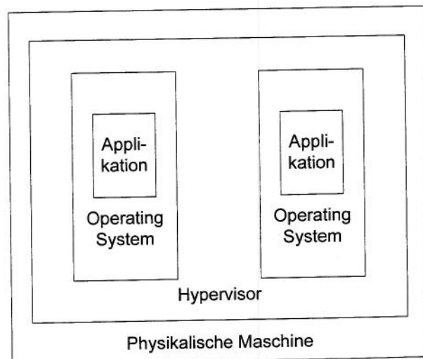
Hypervisor Architektur
